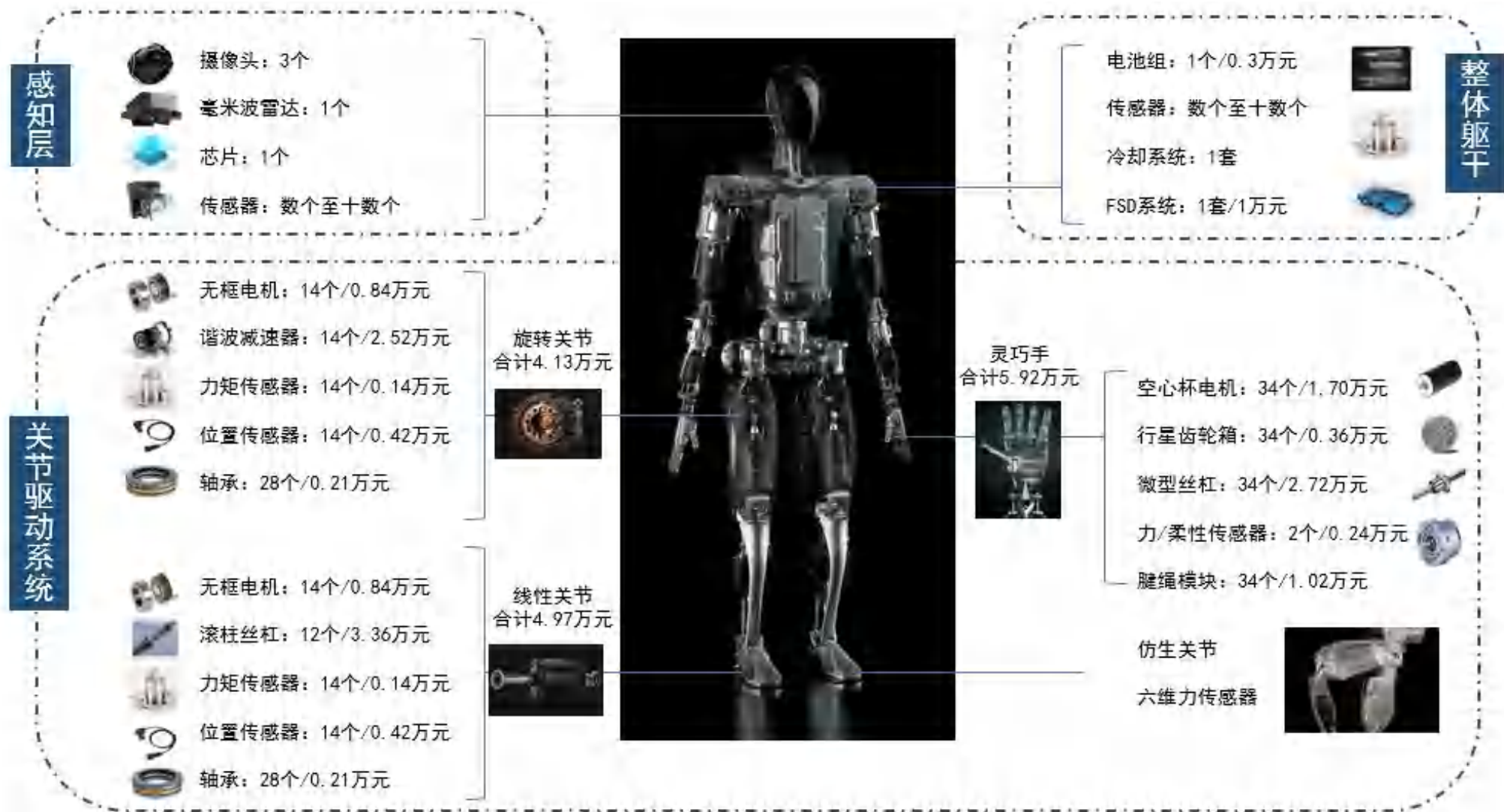
图2：特斯拉人形机器人Optimus结构（以Gen 3为例）
