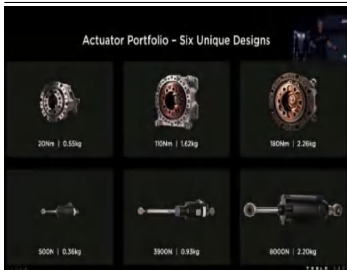
图8：Optimus采用六种标准执行器
