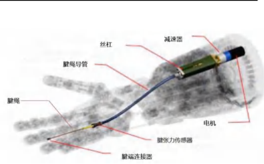
图12：腱绳传动系统工作原理
