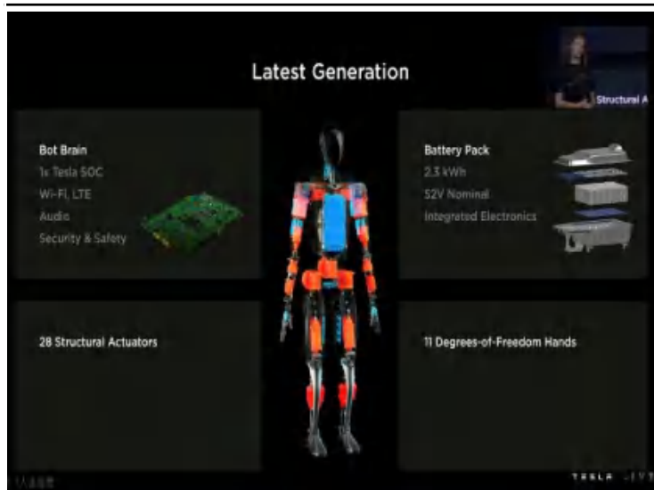
图7：Optimus配备2.3kWh/52V 电池组及SOC芯片
